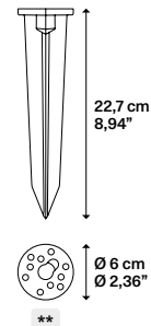
Spike for direct ground installation Picchetto per installazione nel terreno
