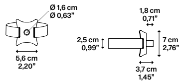
Fixing tree strap (max length 5 m - 196,85") Cinghia di fissaggio per albero (lunghezza max 5 m - 196,85")
